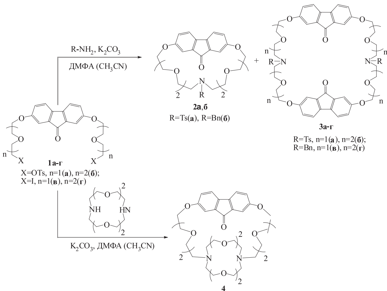
Схема 1. Синтез флуореноноазакраунофанов 2а,б , 3а-г и флуоренонокриптанда 4 .
